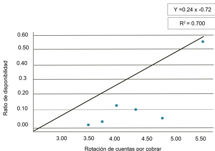
Figura 2 Coeficiente de determinación
